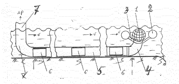
Рис. II-2. Схема размещения трубопровода с включенными последовательно ЭГН.
