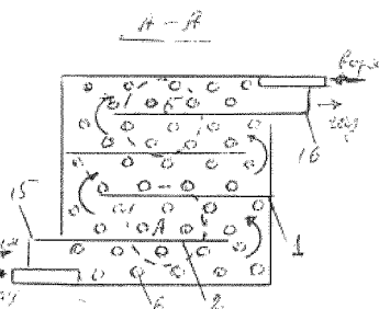
Рис. 2-4. Горизонтальный разрез
