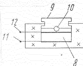
Рис. I-5. Продольный разрез формирователя разрядов электролитического типа (Фиг.4 по источнику 3)
