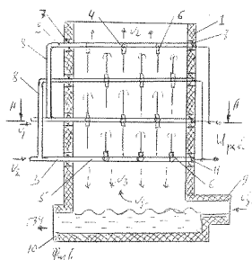
Рис. II-1. Вертикальный разрез фильтра.
