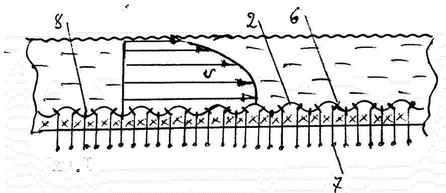
Рис. III-3. Годограф скорости потока по сечению канала. (Фиг. 3 по источнику 6)
