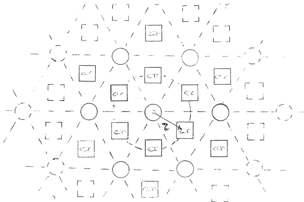
Рис. III-2. План на поверхности земли размещения треугольной ячеистой схемы скважин, образующих ячеистую структуру теплосъема.
