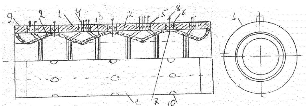
Рис.IV-1. Вид сбоку реверсивного насоса с \frac{1}{4} выреза радиальными плоскостями
