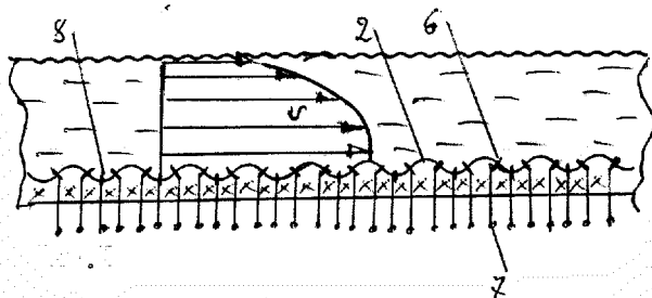
Рис.III-3. Гидрограф скорости потока по сечению канала. (Фиг.3 по источнику 6)
