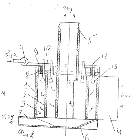
Рис. II-6. Вертикальный разрез ионно-лучевого фильтра
