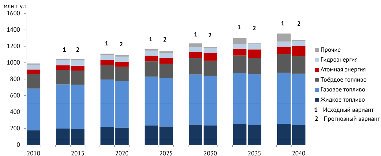
Рисунок 4.2. – Потребление первичных энергоресурсов в России по видам топлива
