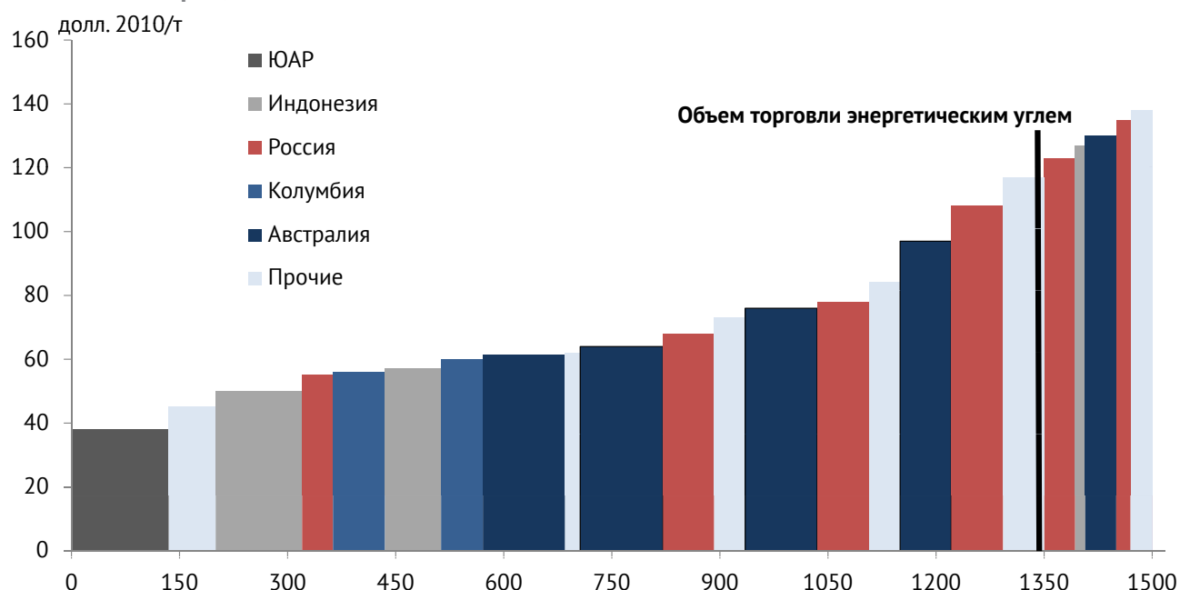
Рисунок 2.37. – Предложение на энергетический уголь в международной торговле, базовый сценарий, 2040г.*
