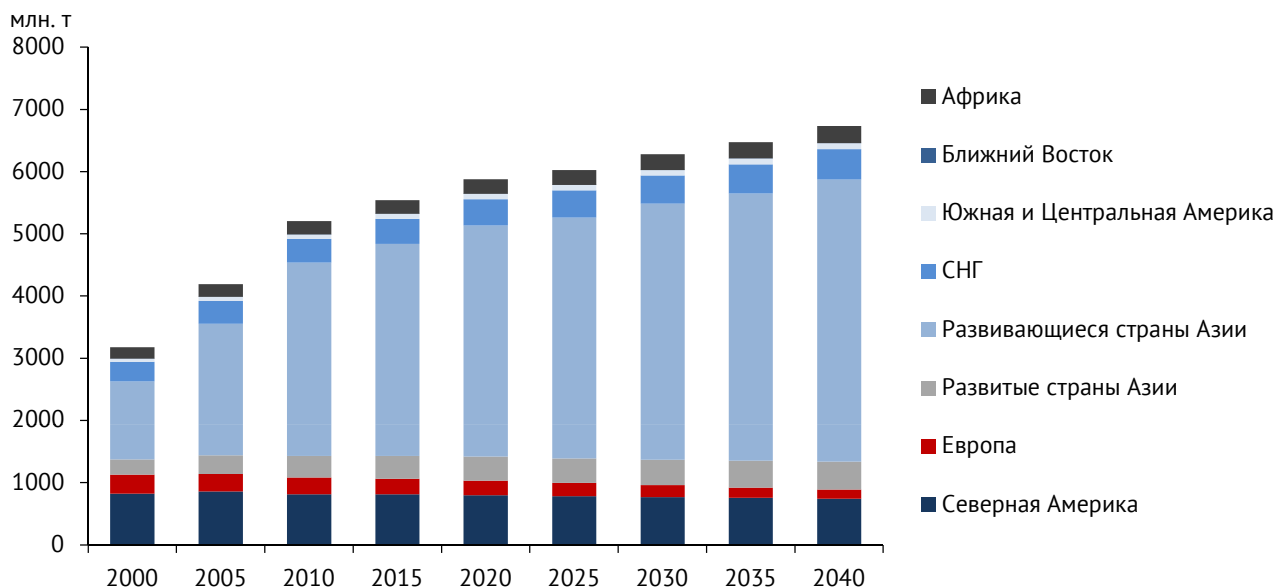
Рисунок 2.36. – Динамика и прогноз добычи угля, базовый сценарий
