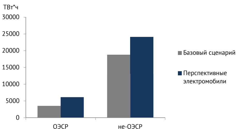
Рисунок 3.21. – Прирост производства электроэнергии по сценариям в 2010–2040 гг.
