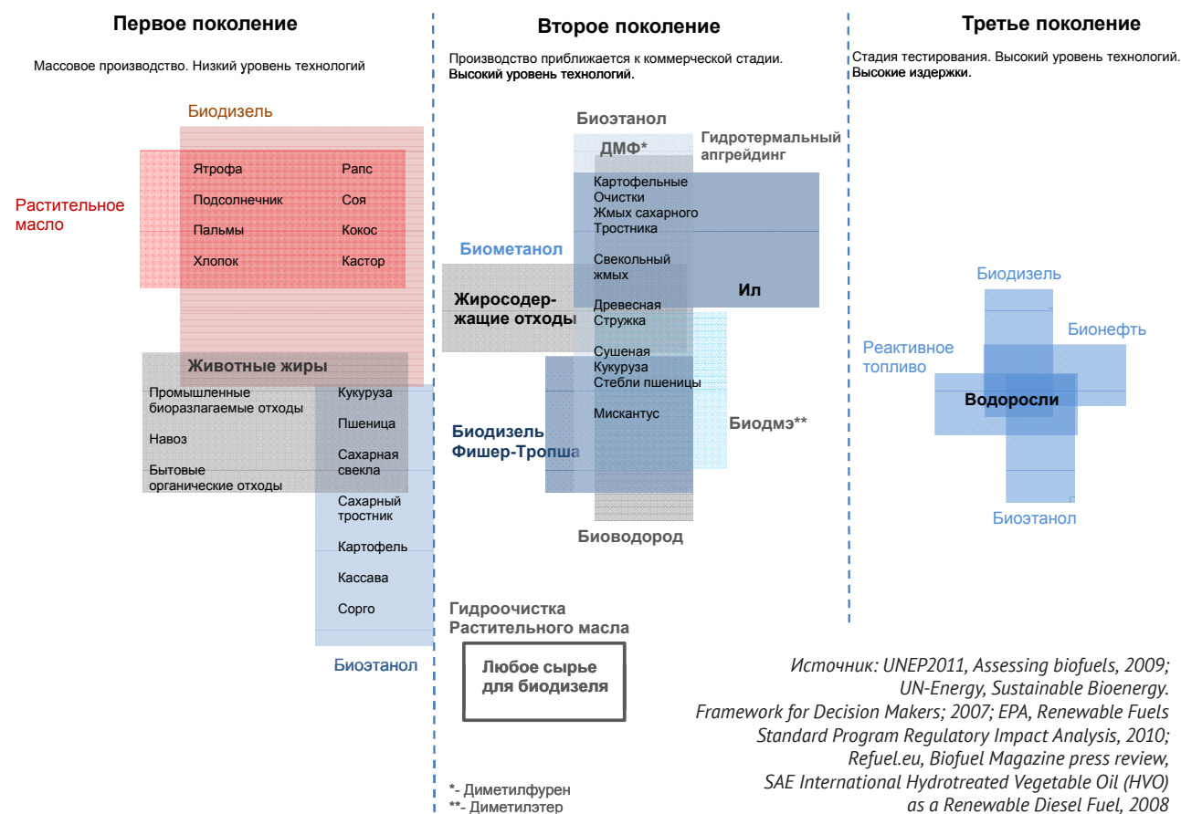
Рисунок 3.18. – Сырье для получения различных видов биотоплива
