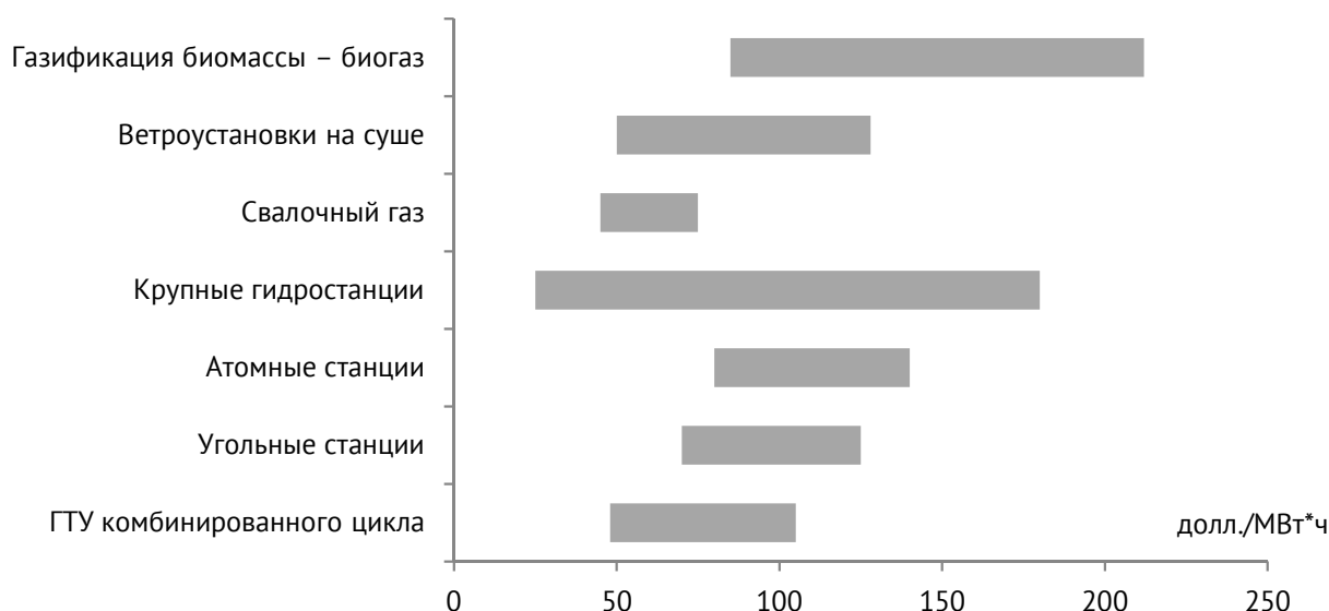
Рисунок 3.25 – Удельные дисконтированные затраты производства электроэнергии по видам энергоресурсов
