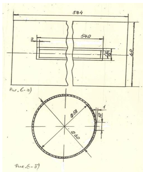
Рис.7 Рабочая камера насоса ( Рис.6 по источнику /3/ )
