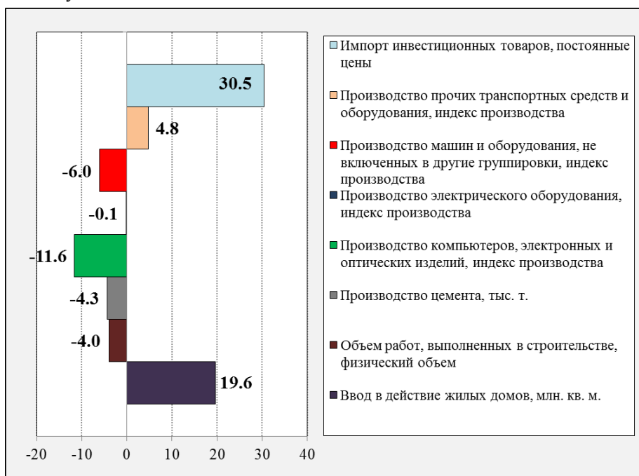
Рис.2. Косвенные показатели инвестиционной активности в экономике январь-декабрь 2017 г., темп прироста к январю-декабрю 2016г.
