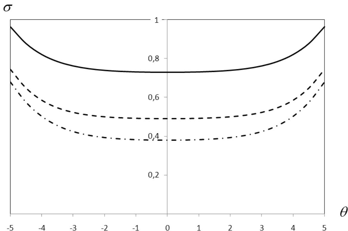
Рис.4. Зависимость стандартной ошибки измерения от уровня подготовленности: ————— - тест из дихотомических заданий; - - - - - тест из политомических заданий, оцениваемых двумя баллами; - · - · - · - тест из политомических заданий, оцениваемых тремя баллами
