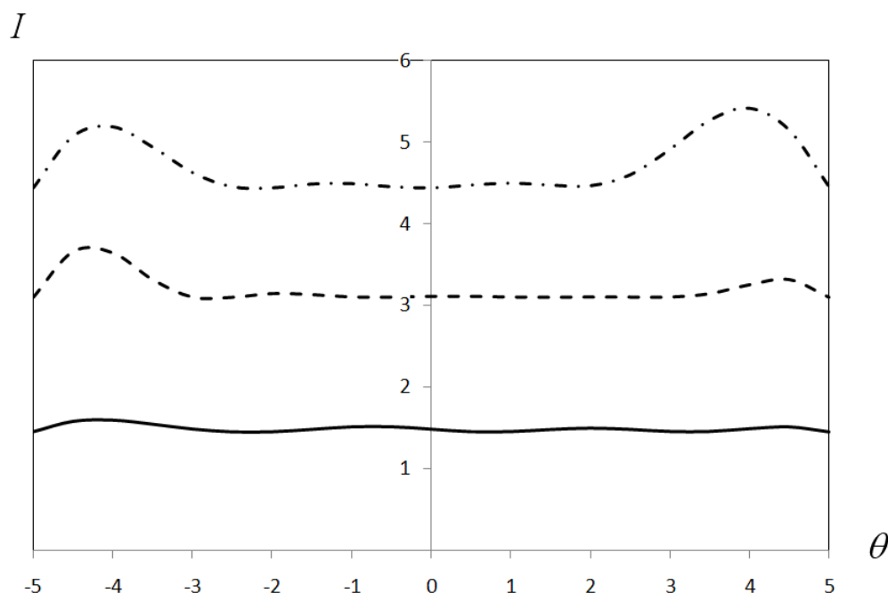
Рис.6. Зависимость стандартной ошибки измерения от уровня подготовленности испытуемого: ———— - тест из дихотомических заданий; - - - - - тест из политомических заданий, оцениваемых двумя баллами; - · - · - · - тест из политомических заданий, оцениваемых тремя баллами
