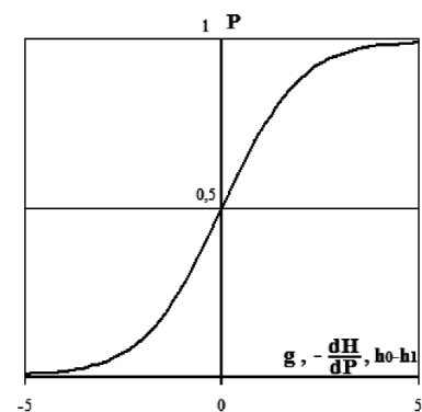
Рис. 2. Логистическая кривая с различными осями абсцисс
