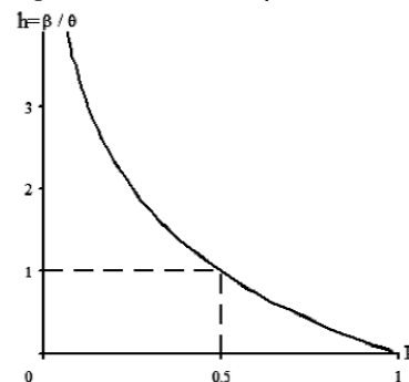
Рис. 7. График функции частной энтропии h(P)
