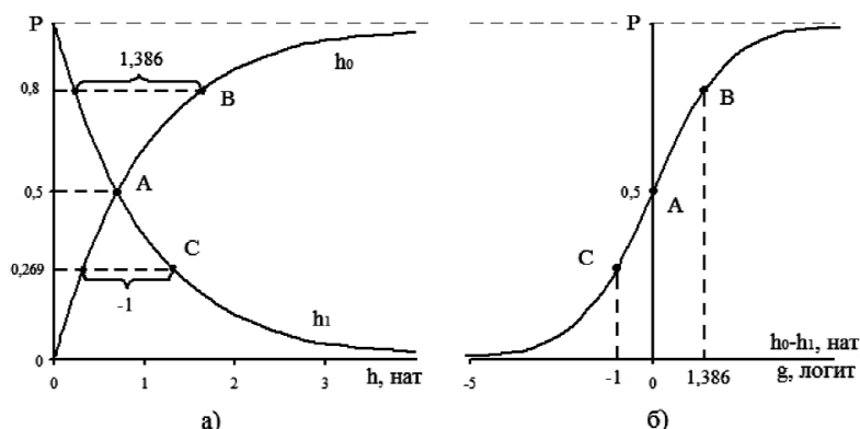
Рис. 3. Информационная трактовка модели Раша: частная энтропия h
