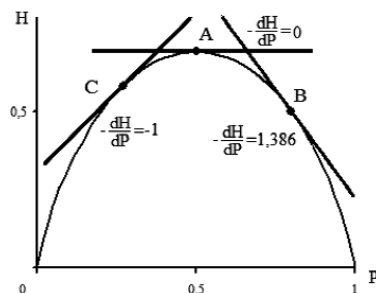
Рис. 3в. Информационная трактовка модели Раша: средняя энтропия H
