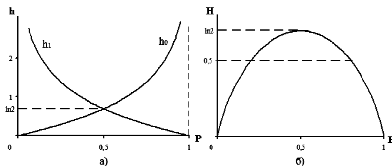
Рис. 1. Графики функций энтропий h(x) и H(x)
