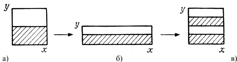
Рис. 23. Последовательные итерации преобразования пекаря приводят к фрагментированию заштрихованных и светлых полосок на все большее и большее число разъединенных областей
