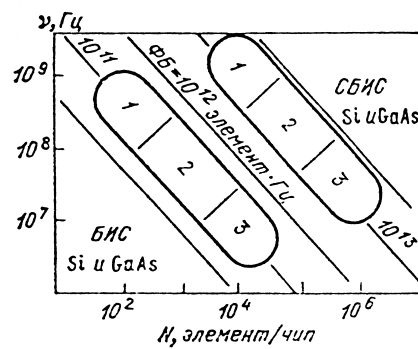
Рис. 33. Характеристики развития СБИС: 1 — ИС для управления и вычисления; 2 — радиолокационный цифровой процессор; 3 — чувствительный сигнальный процессор (Значения ФБ области применения)
