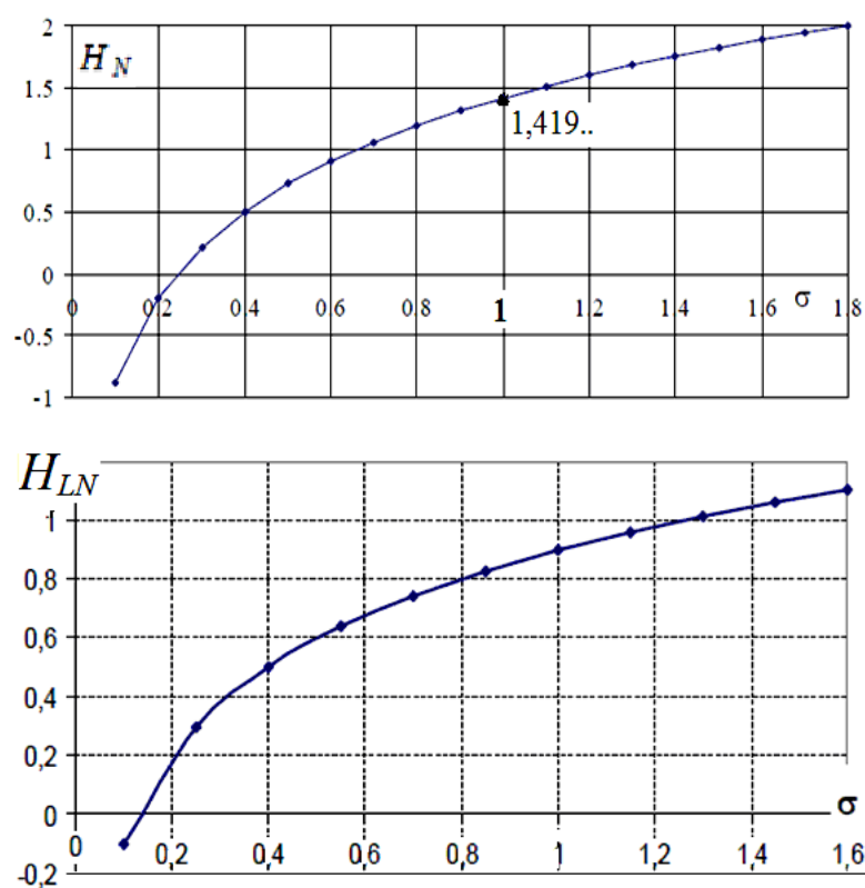
Рис. 14. Зависимость дифференциальной энтропии H_N нормального и H_{LN} логнормального распределения от параметра \sigma , превратившегося в параметр формы H_{LN}
