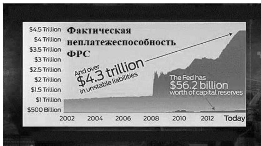
Рисунок 5 – Разрыв между обязательствами и капиталом ФРС США.
