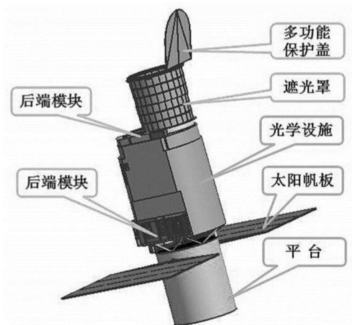
图 13 多功能主动光学设施示意图
