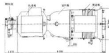
“神舟”飞船发射状态外型图
