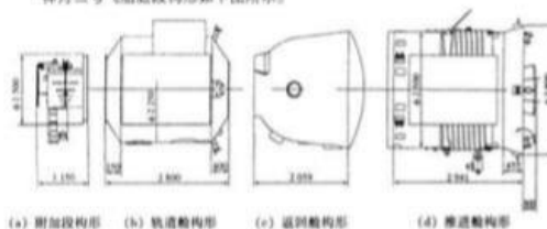
“神舟”飞船发射状态外型图
